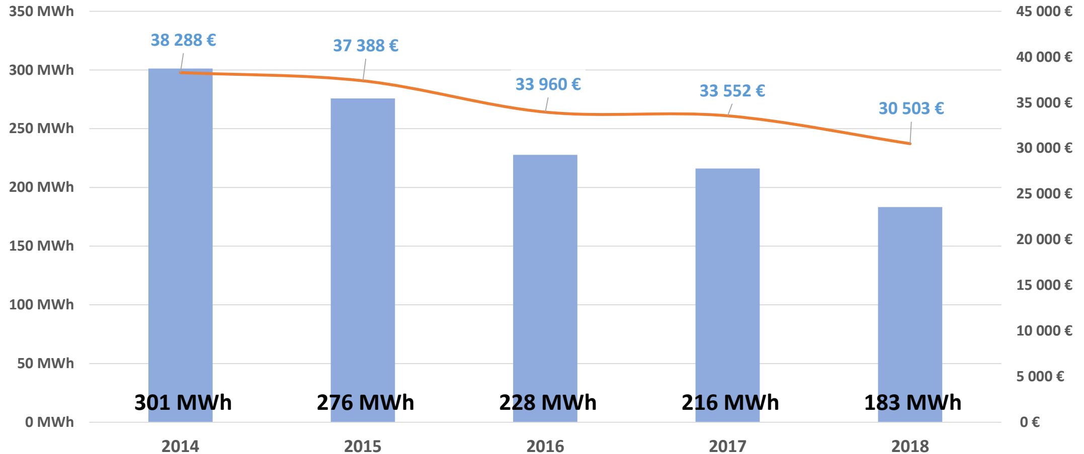
Evolution des consommations et dépenses de l'éclairage public
